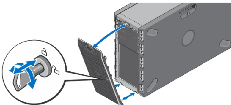
Figure 5. Installation du cadre
