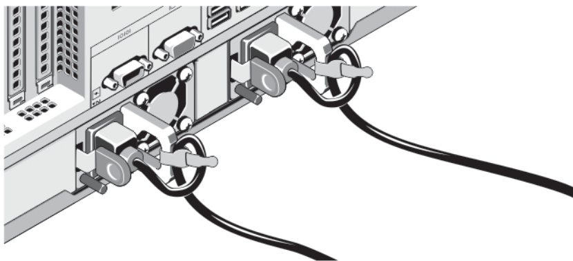
Figure 3. Fixation du ou des câbles d'alimentation
